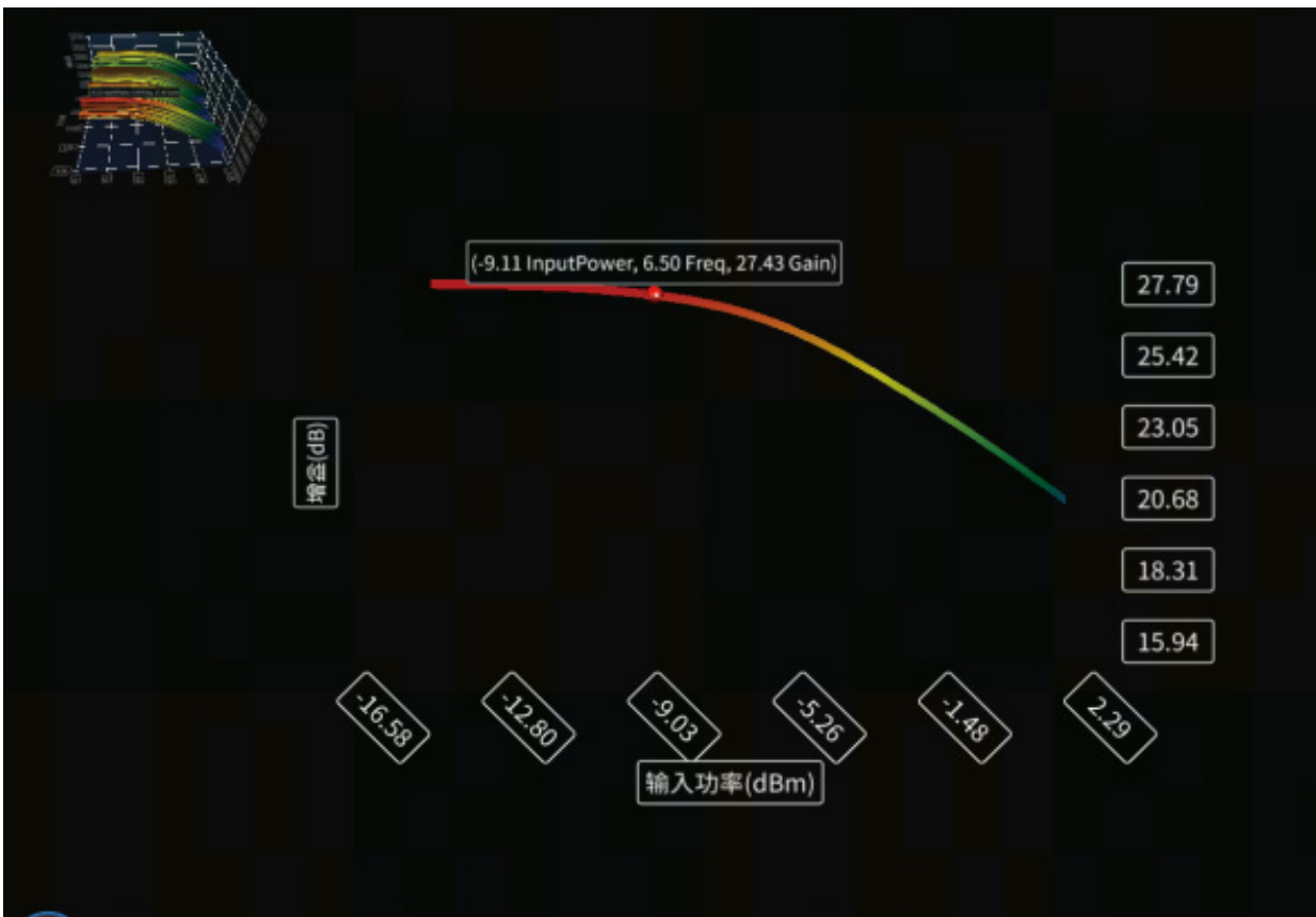
频率切面
