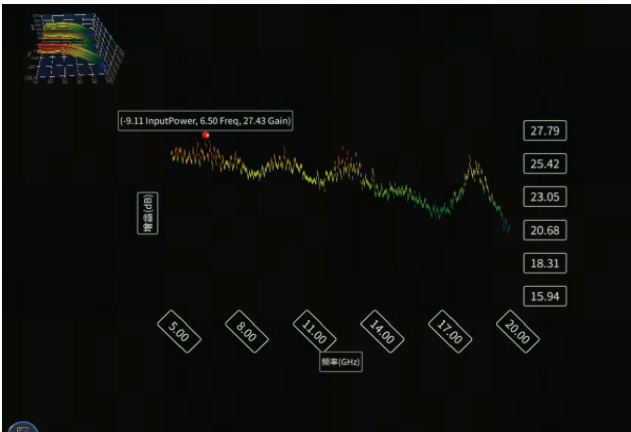
功率切面
