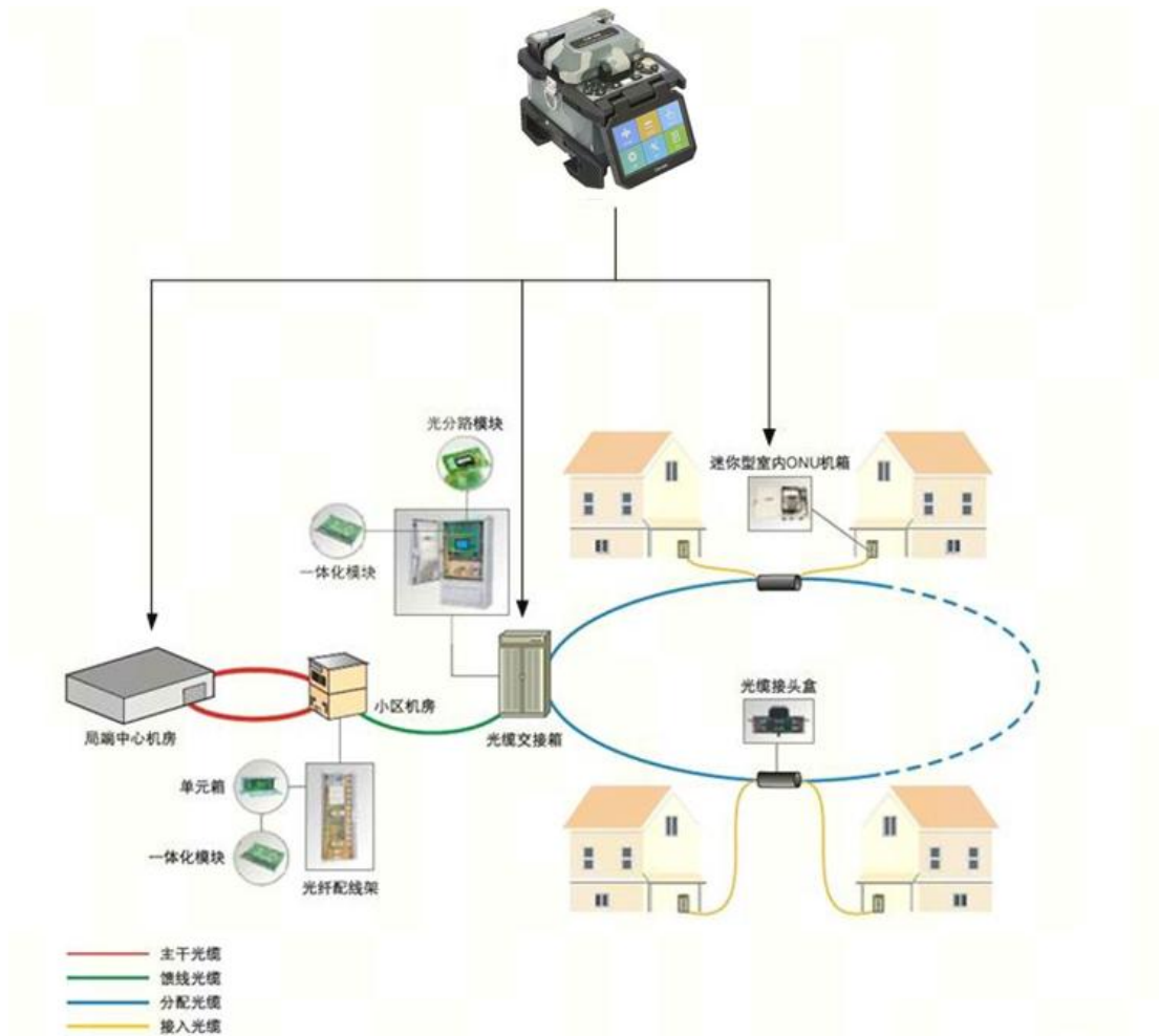
6481 系列光纤熔接机典型应用
