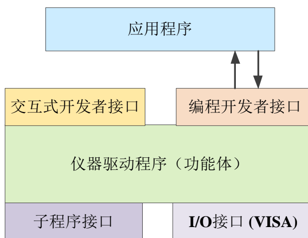
图 9.9 仪器驱动器结构模型
