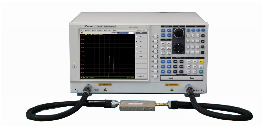
附图 1.4 滤波器测试连接图
