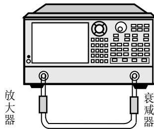
图 8.17 绝对输出功率测量连接
