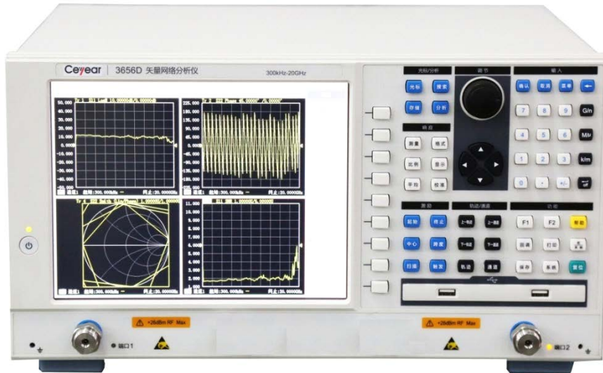
图 3.3 3656 前面板
