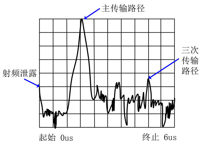
附图 2.16 带通模式下的传输测量
