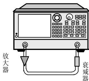
图 8.22 小信号增益和平坦度测量连接
