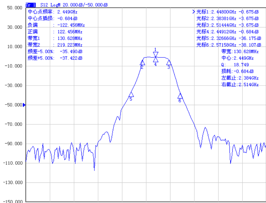
图 3.48 滤波器测试
