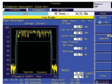
脉冲波形显示 (8PSK)
