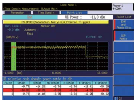
码域功率
