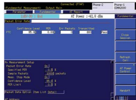
PER
