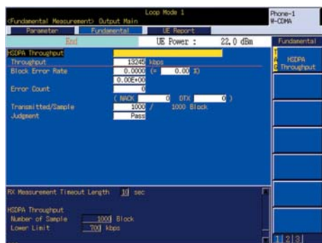
吞吐量监测
